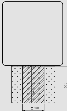
Einfundamentierung des Terrasoft Zylinders mit Hilfe des Bodenankers.
