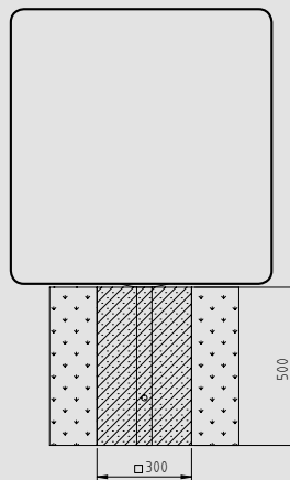
Einfundamentierung des Terrasoft-Polygons mit Hilfe des Bodenankers.
