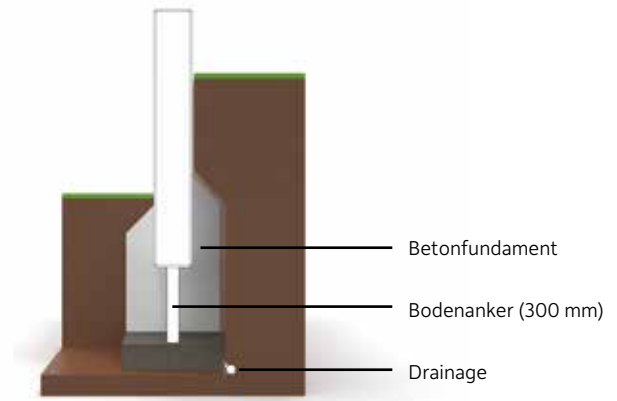
Einbau der Palisade im Betonfundament mit rückseitiger Abstützung und Drainage
