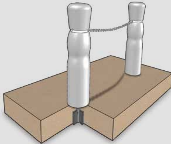
Einfundamentierung des Begrenzungspfostens mit Hilfe des Bodenankers auf losem Untergrund.
